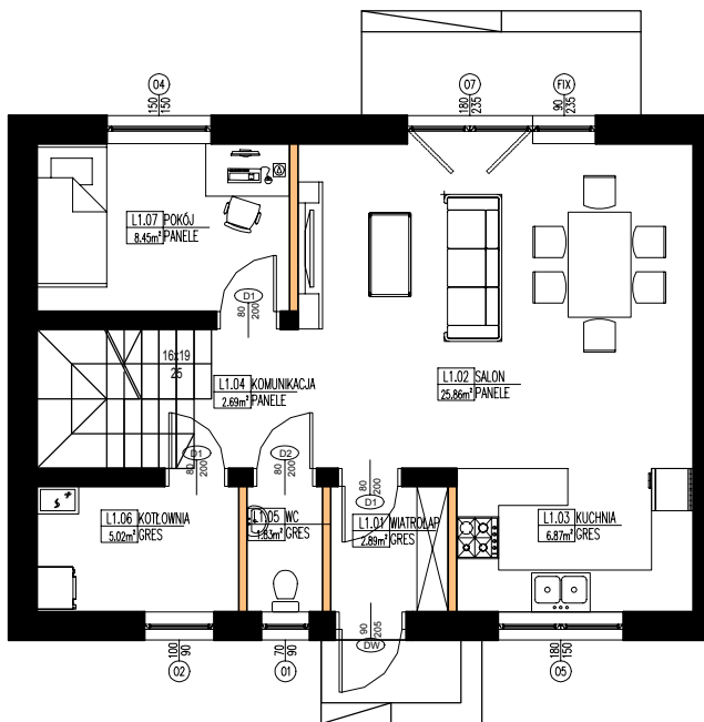
RZUT PARTERU
