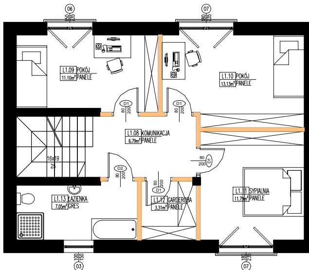
RZUT PIĘTRA
