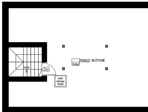
RZUT PODDASZA
