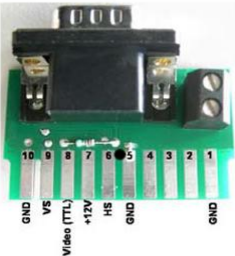
Podłączenie monitora mono
