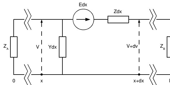
Rys.1. Obwód zastępczy rurociągu pod wpływem oddziaływania indukcyjnego.
