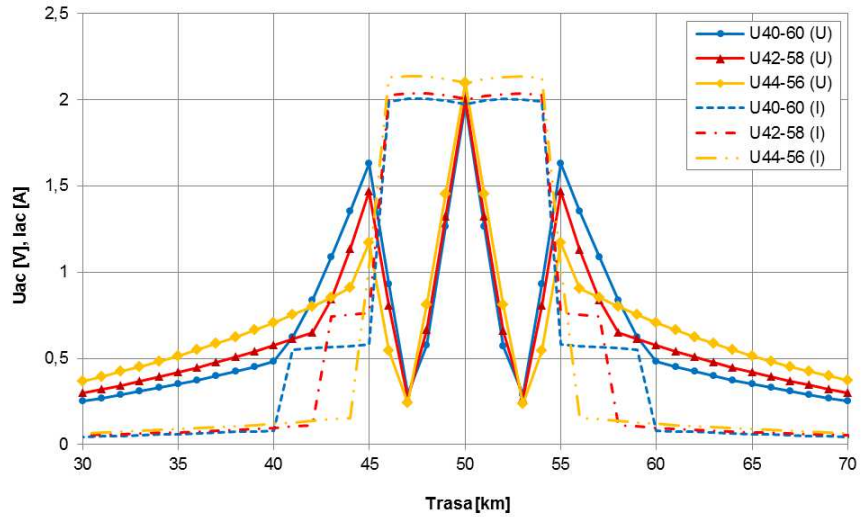
Rys.11. Uzamienia obu sekcji na 40,45,50,55 i 60km, 42,45,50,55 i 58km, 44,45,50,55 i 56km.
