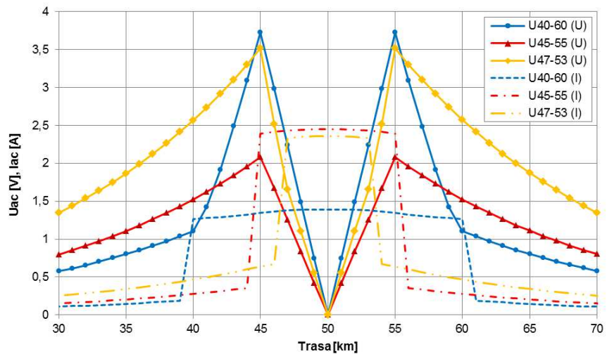
Rys.6. Uziemia na 40 i 60km, 45 i 55km, 47 i 53km (rezystancja 1Ω).
