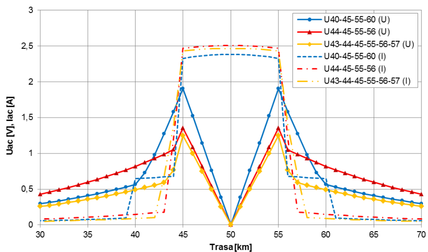
Rys.7. Uziemienia na 40,45,55 i 60km, 44,45,55 i 56km, 43,44,45,55,56 i 57km (rezystancja 1\Omega ).
