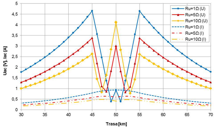
Rys.9. Uziemienia obu sekcji na 50km (różne rezystancje).
