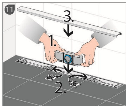
11 1. Sifon opnieuw in de drain steken. 2. I-Cube houders opnieuw in het rooster steken. 3. Het sierprofiel terug in het rooster plaatsen.
