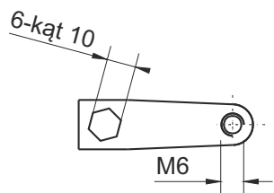
Dźwignia na wałek łącznika pomocniczego
